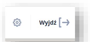
Rys. 12. Ikona USTAWIENIA
